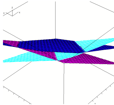
je zwei Ebenen schneiden sich: drei Schnittgeraden
