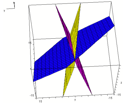
alle drei Ebenen schneiden sich in einer Geraden
