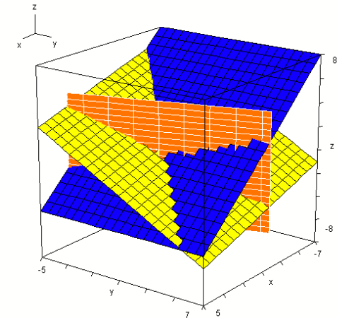
alle drei Ebenen schneiden sich in einem Punkt
