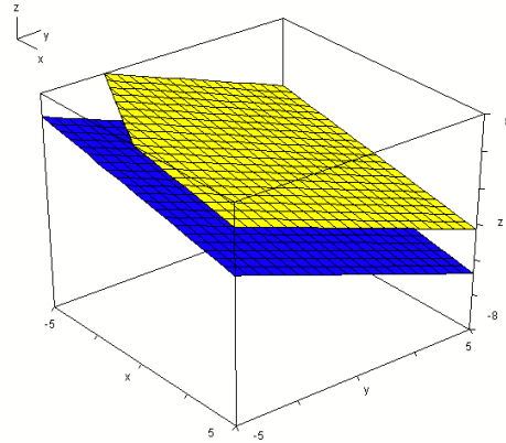
zwei Ebenen identisch, die dritte parallel
