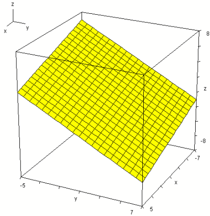
alle drei Ebenen identisch
