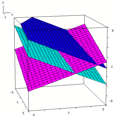
zwei Ebenen parallel, die dritte schneidet beide: zwei Schnittgeraden
