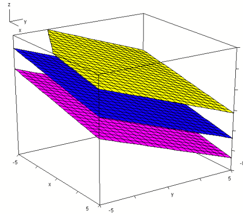
alle drei Ebenen parallel
