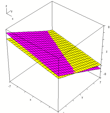
zwei Ebenen identisch, die dritte schneidet
